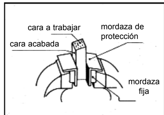
Fig. 33: mordaza de protección
