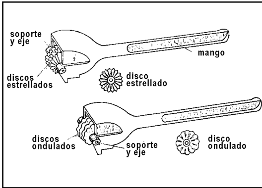
Fig. 49. Rectificadores
