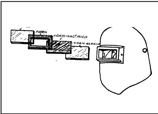
Fig. 79: Visores
