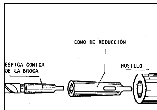
Fig. 43. Cono
