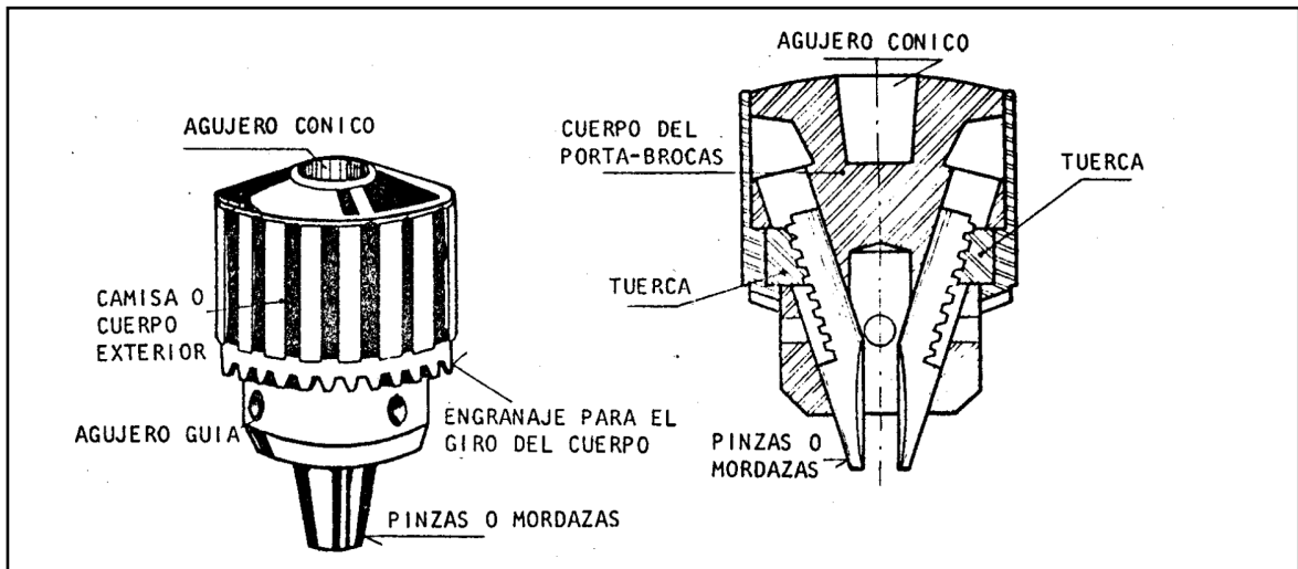
Fig. 40. mandril (corte)
