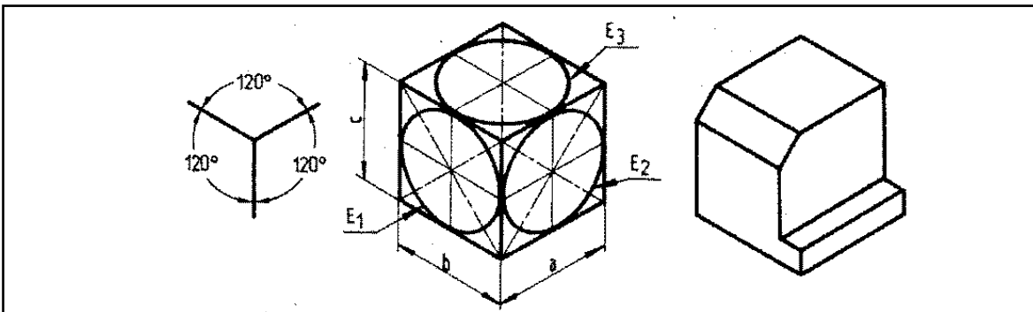
Fig 62: Perspectiva isométrica
