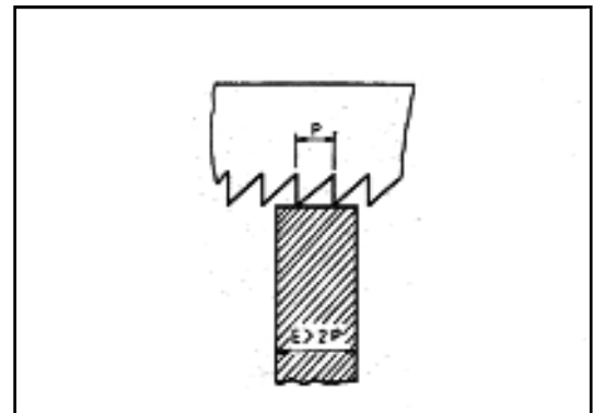
Fig. 23: pasos de dientes
