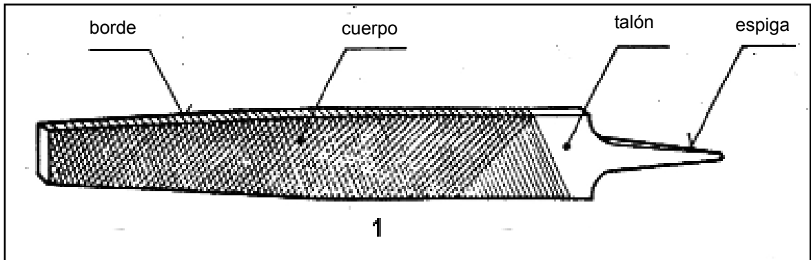
Fig. 5 La lima
